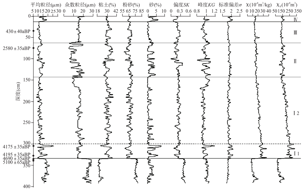
图 2 SC7 孔各粒度参数与磁化率垂向变化
