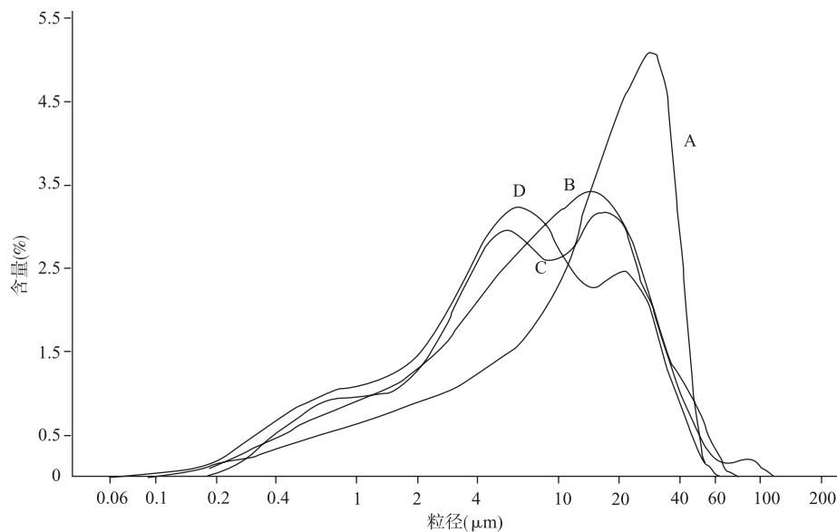
图 3 SC7 柱样沉积物粒度频率分布曲线
