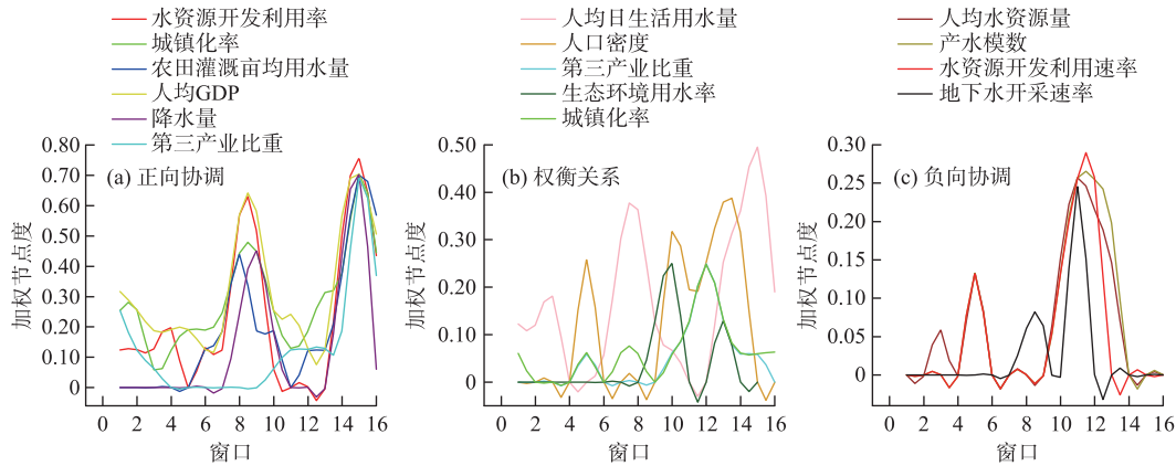
图3 3种耦合关系中的关键指标的加权节点度随窗口的变化 (图中仅显示正向协调关系中最大加权节点度 >0.65 的指标,权衡关系中最大加权节点度 >0.24 的指标和负向协调关系中最大加权节点度 >0.20 的指标)
