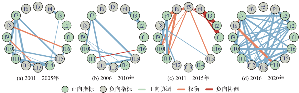
图1 甘肃省水资源承载力系统交互网络
