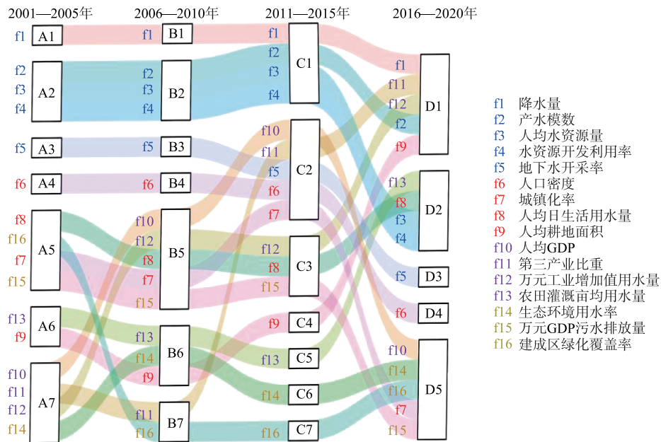
图4 4个阶段下水资源承载力系统的模块化结构(蓝色指标所属水资源子系统,红色指标所属社会子系统,紫色指标所属经济子系统,黄色指标所属生态环境子系统)
