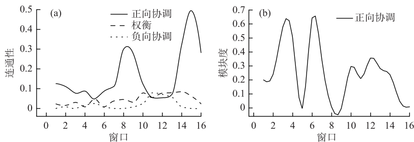
图2 3种耦合关系的连通性(a)和正向协调关系的模块度(b)随窗口的变化
