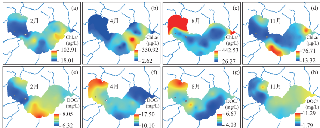
图 3 巢湖表层水体叶绿素 a 和溶解性有机碳浓度的空间分布
