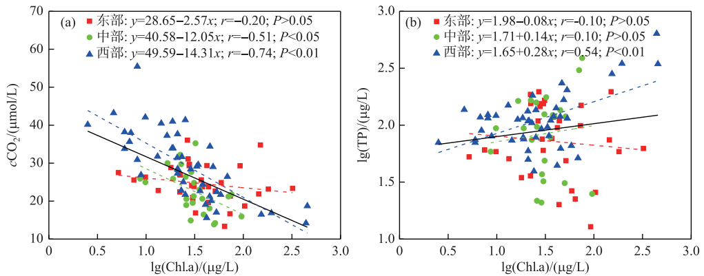
图 6 叶绿素 a 浓度与 \text{CO}_2 浓度(a)和总磷浓度(b)的关系
