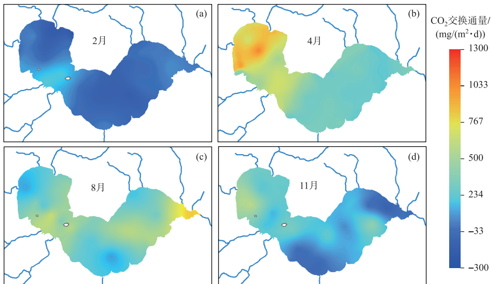
图5 巢湖水—气界面 CO 2 交换通量时空变化
