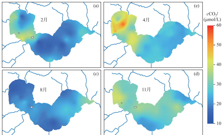
图 4 巢湖表层水体 CO 2 浓度的时空变化
