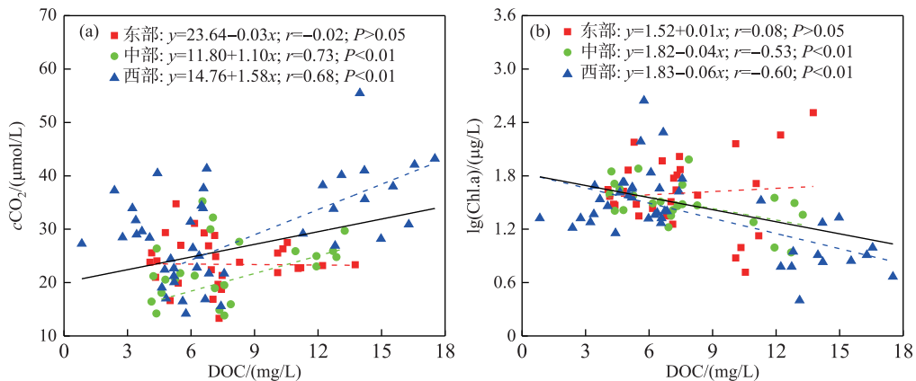
图 7 溶解性有机碳浓度与 \text{CO}_2 浓度(a)和叶绿素 a 浓度(b)的关系
