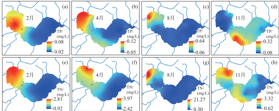
图 2 巢湖表层水体总磷和总氮浓度的空间分布
