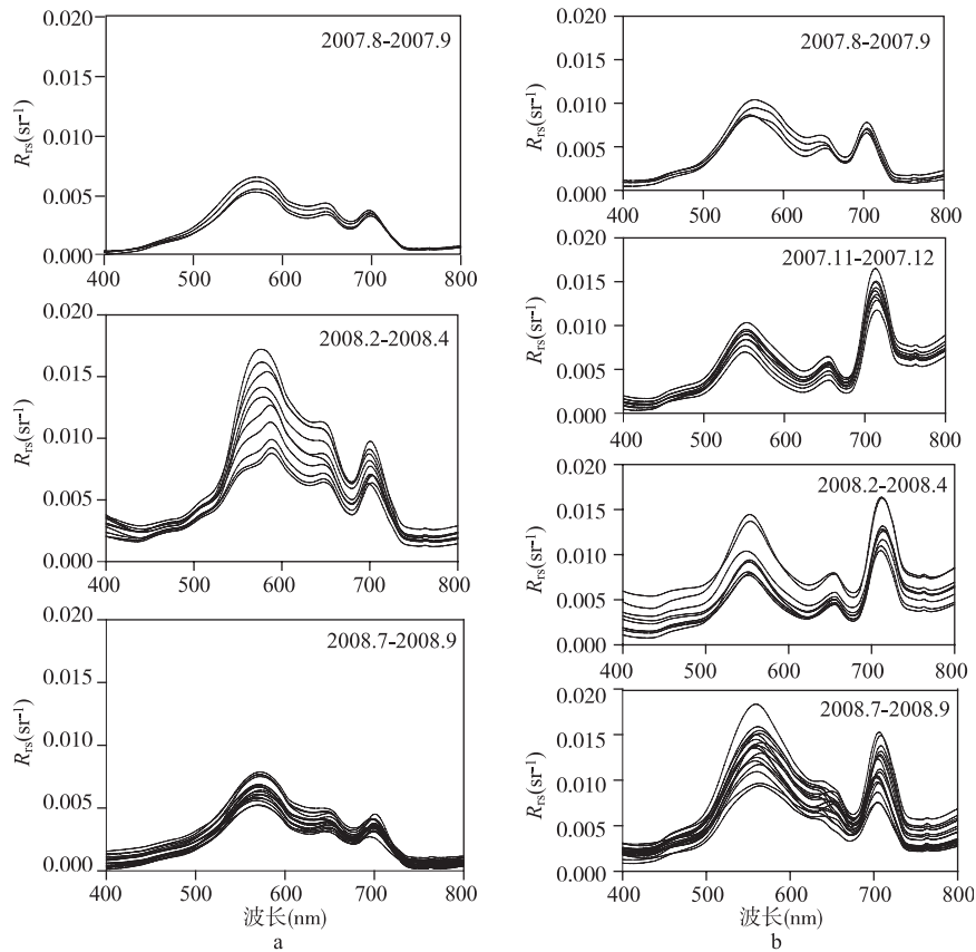
图2 遥感反射率光谱: 水库(a); 芙蓉湖(b)
