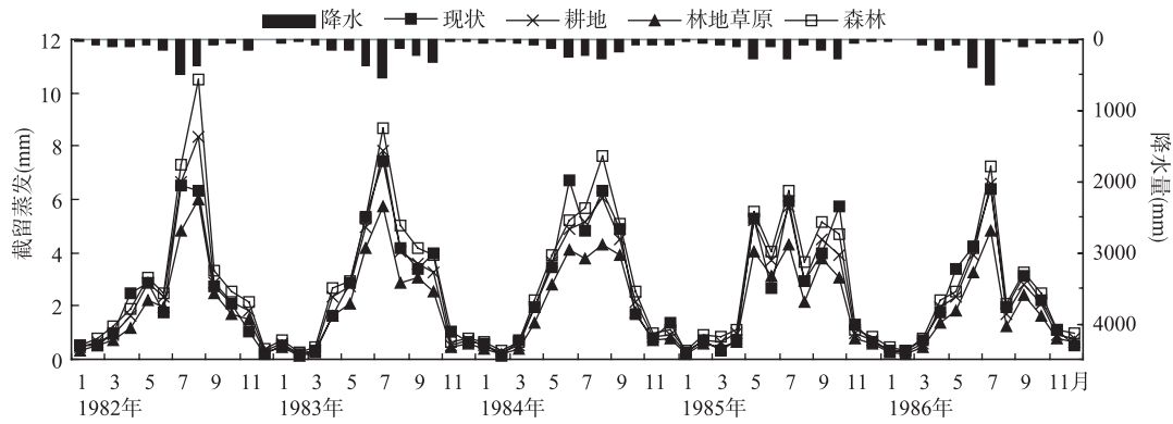
图1 黄泥庄集水区1982-1986年各土地覆被情景下的月截留蒸发量比较
