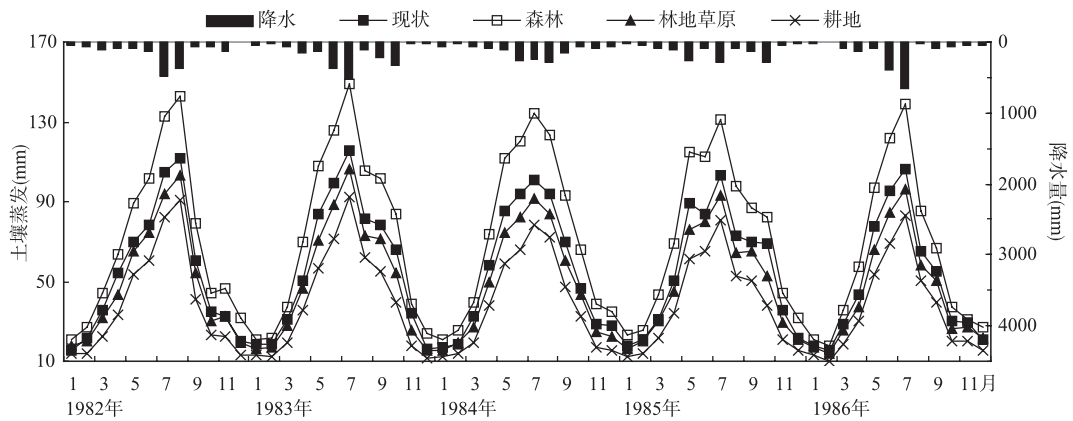
图2 黄泥庄集水区1982-1986年各土地覆被变化情景下的月土壤蒸发量比较
