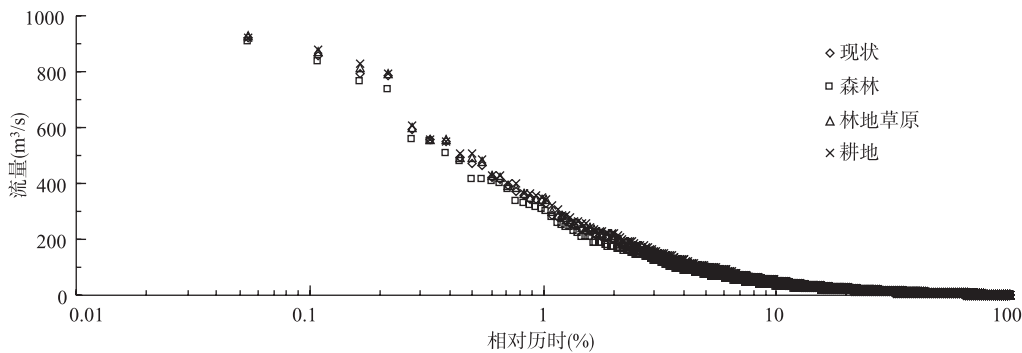
图3 各土地覆被变化情景下黄泥庄集水区1982-1986年日流量历时曲线
