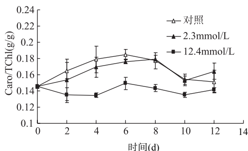
图3 碱度对蛋白核小球藻Caro/Tchl的影响
