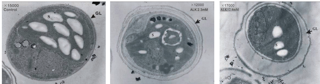
图5 不同碱度条件下培养的蛋白核小球藻的胞外多糖变化
