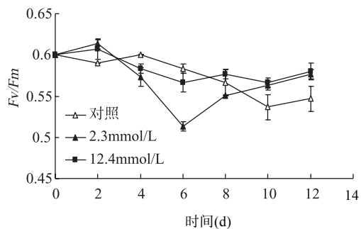
图1 不同碱度下蛋白核小球藻的 F_v/F_m 变化
