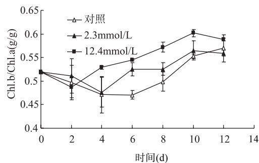
图2 碱度对蛋白核小球藻Chl.b/Chl.a的影响
