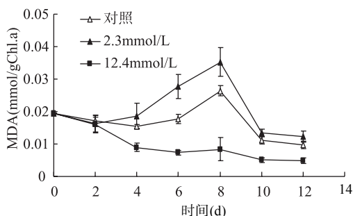
图4 不同碱度下蛋白核小球藻的MDA含量变化
