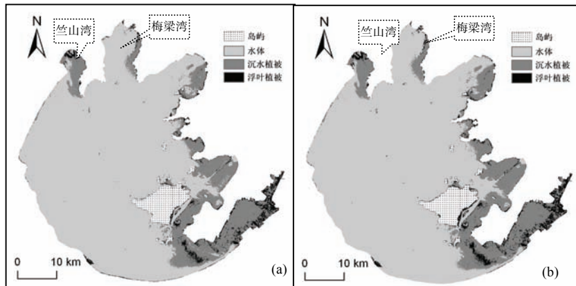
图 6 水体透明度参与的太湖水生植被分类(水体、以沉水植被为主导的水生植被类、以浮叶植被为主导的水生植被类): (a)利用 RVI 的分类结果; (b)利用 NDVI 分类结果
