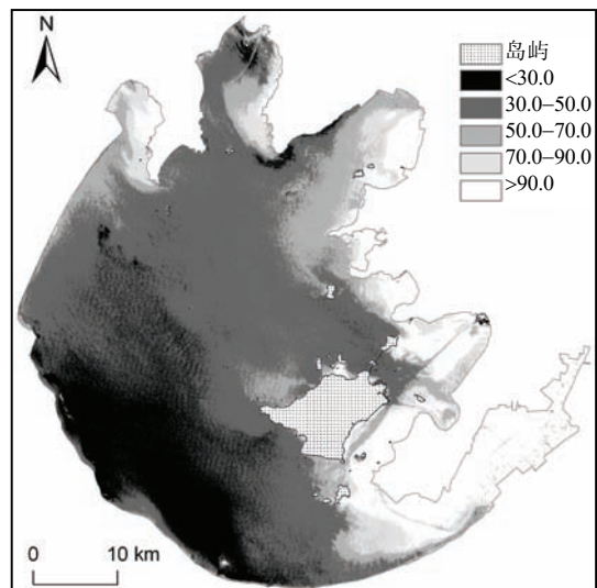
图 2 2002 年 7 月 15 日太湖透明度的空间分布
