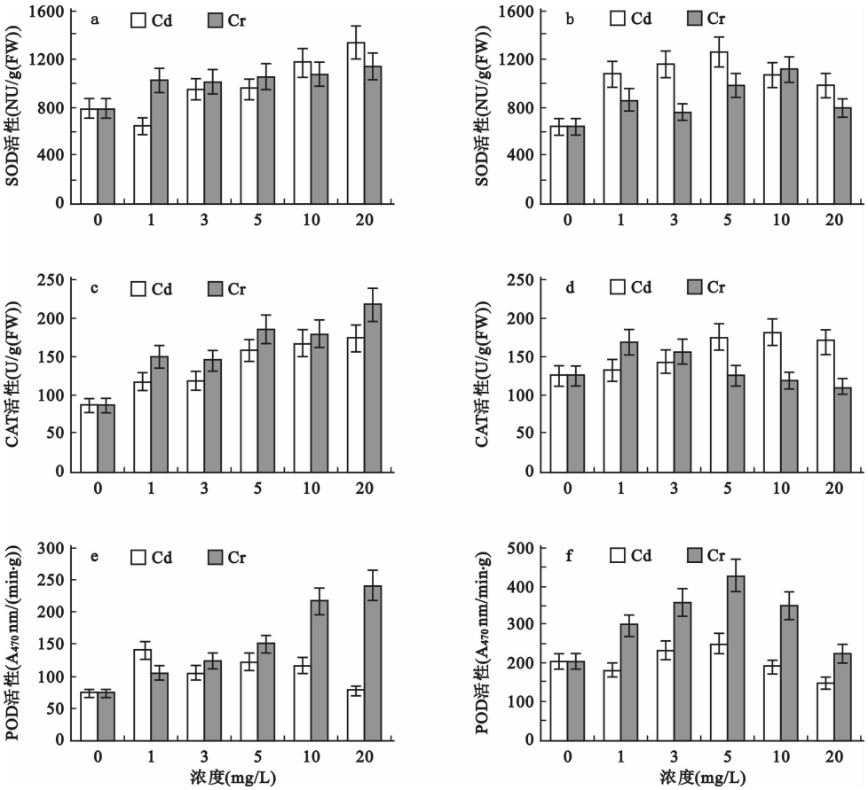
图3 Cd 2+ 和Cr 6+ 对慈菇根及叶中抗氧化酶活性的影响
