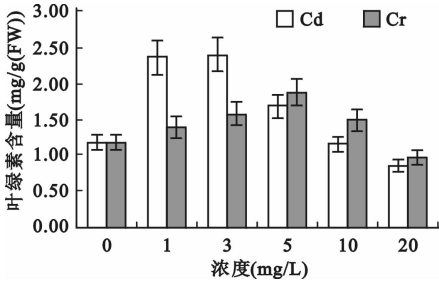
图 1 Cd 2+ 和 Cr 6+ 对慈姑叶绿素含量的影响
