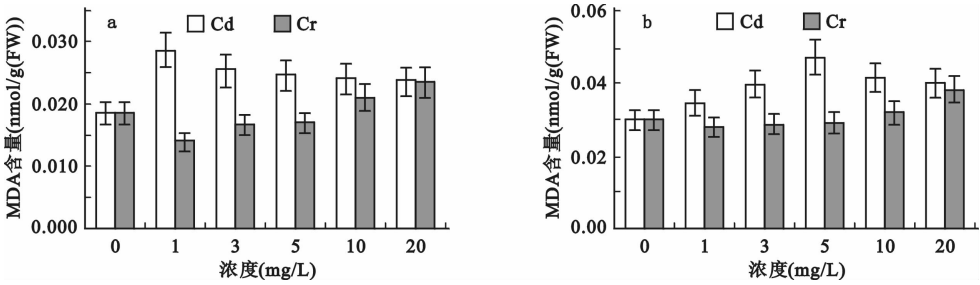
图5 Cd 2+ 和 Cr 6+ 对慈姑根(a)和叶(b)中 MDA 含量的影响
