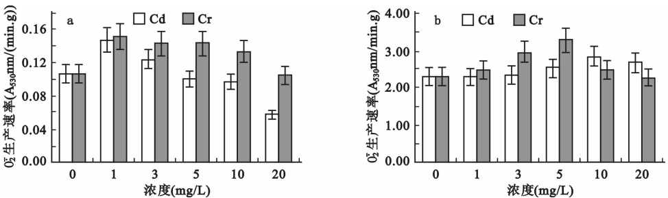
图4 Cd 2+ 和Cr 6+ 对慈菇根(a)和叶(b)中超氧阴离子产生速率的影响
