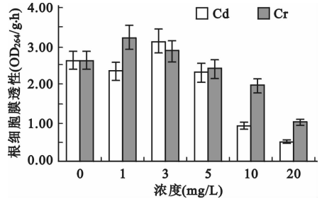
图 2 Cd 2+ 和 Cr 6+ 对慈姑根细胞膜透性的影响
