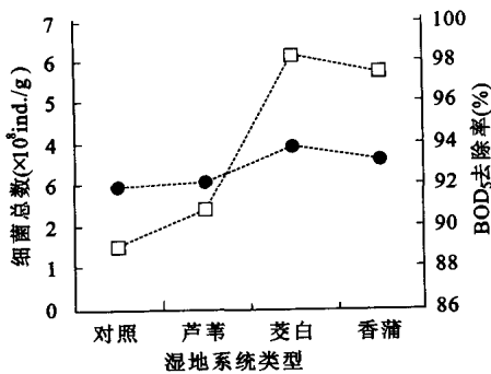
图 1 实验湿地小试系统夏季根区细菌总数与 BOD 5 去除率的相关性
