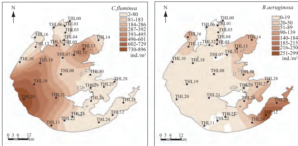
图 3 太湖河蚬、铜锈环棱螺空间分布格局图
