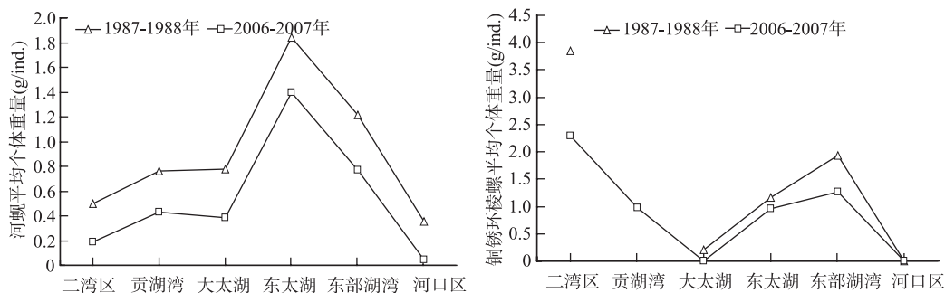
图 4 20 年来河蚬、铜锈环棱螺单位个体重量变化
