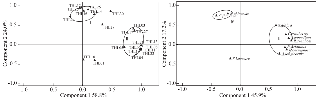
图 2 太湖软体动物主成分分析
