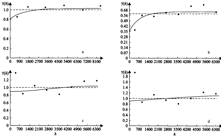
图3 百花湖表层水中不同形态汞含量的半变异函数(a. 溶解态汞; b. 活性汞; c. 颗粒态汞; d. 总汞)
