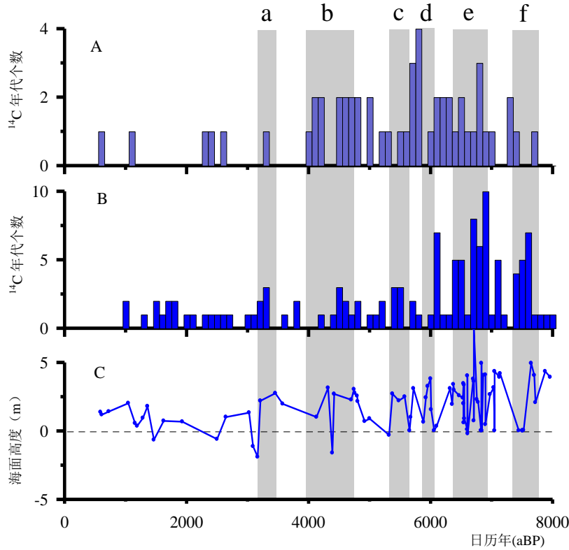
图1 长江三角洲地区埋藏古树(A)、泥炭(B)、全新世海面(C)变化比较
