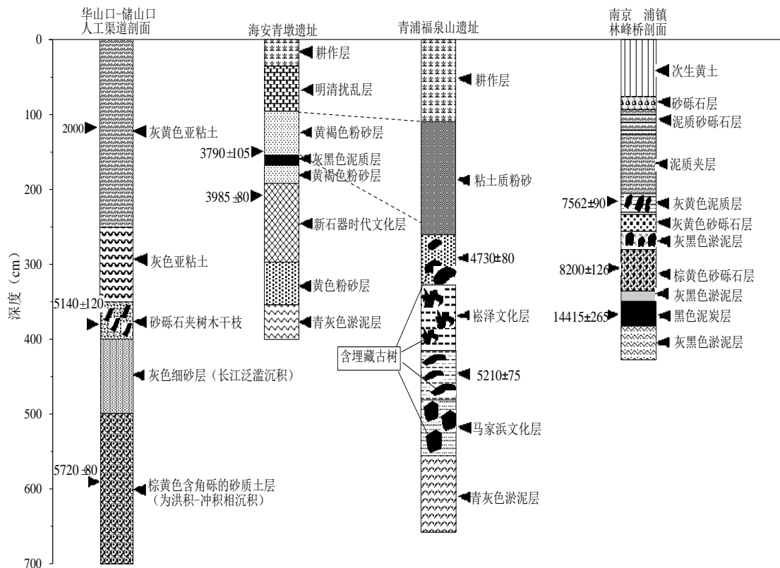
图2 长江三角洲地区自然沉积剖面与新石器时代考古遗址剖面对比示意图 [23-26]
