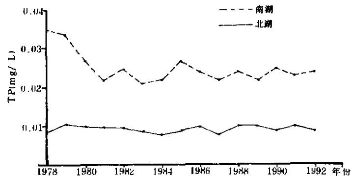
图 1 日本琵琶湖总磷历年变化
